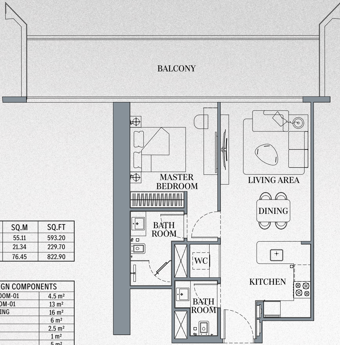
1 Bedroom Unit - Type 2
